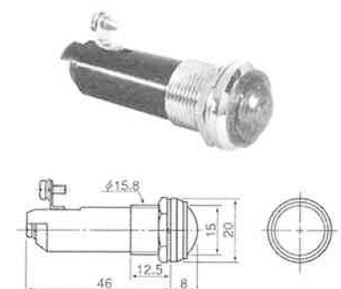
■BT-16HBB形 AC/DC110V, 24V 〈文字彫刻可〉
