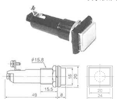
■BT-16HKB形 AC/DC110V, 24V 〈文字彫刻可〉
