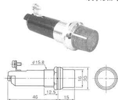
■BT-16H形 AC/DC110V, 24V 〈文字彫刻可〉
