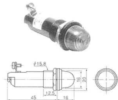
■BT-16HM形 AC/DC110V, 24V
