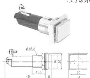
■BT-16HK形 AC/DC110V, 24V 〈文字彫刻可〉
