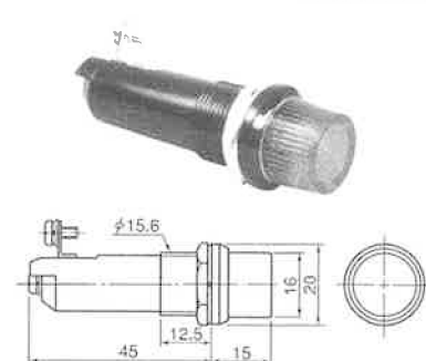
■BT-16HB形 AC/DC110V, 24V 〈文字彫刻可〉
