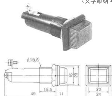
■BT-16NKB形 AC/DC110V, 4V 〈文字彫刻可〉
