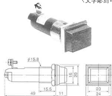
■BT-16NK形 AC/DC110V, 24V 〈文字彫刻可〉
