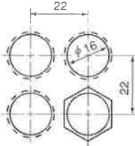
ナット二面幅 18mm
