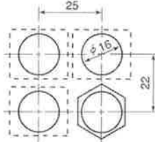
ナット二面幅 18mm
