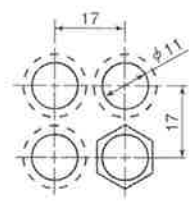
ナット二面幅 19mm
