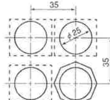
ナット二面幅 31mm
