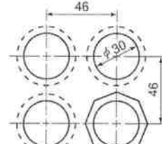
ナット二面幅 38mm
