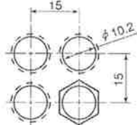
ナット二面幅 12mm
