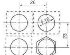
ナット二面幅 18mm
