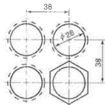
ナット二面幅33mm
