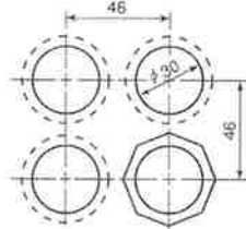
ナット二面幅38mm (八角ナット)
