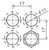
ナット二面幅13mm
