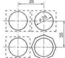
ナット二面幅31mm
