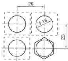
ナット二面幅19mm
