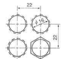
ナット二面幅19mm
