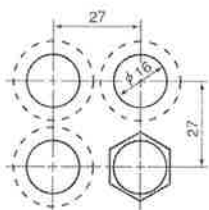
ナット二面幅18mm
